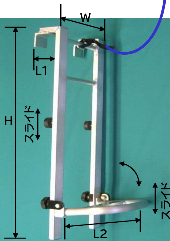
落下防止のワンタッチベルト付
